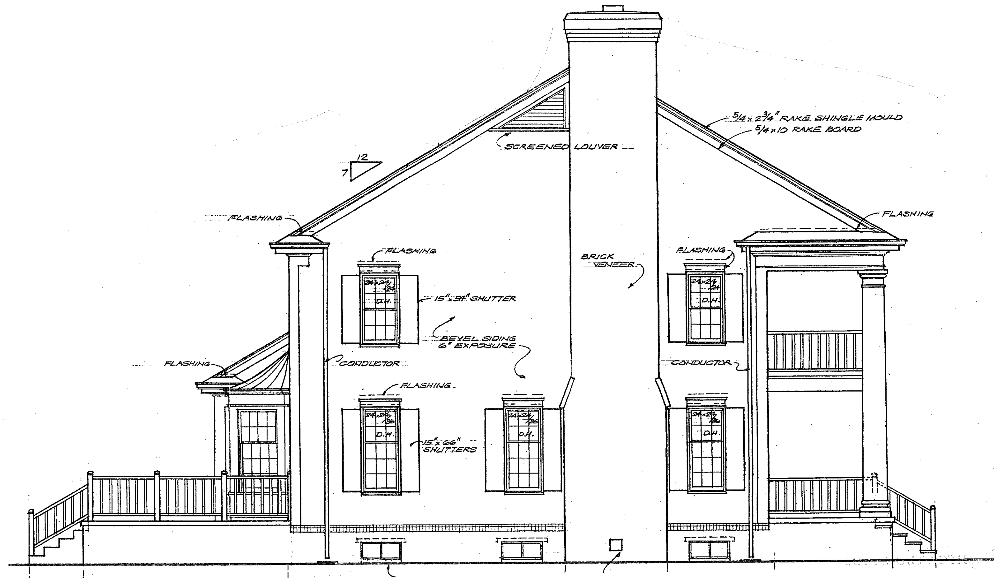
LEFT SIDE ELEV.
