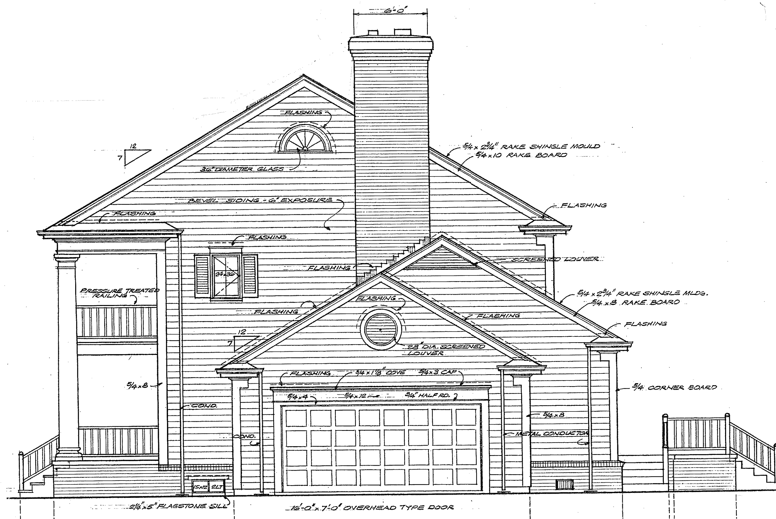
RIGHT SIDE ELEV.
